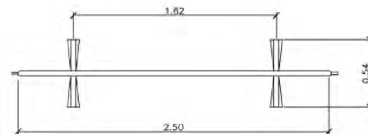
VALLA MÓVIL DE PROTECCIÓN Y PROHIBICIÓN DE PASO
