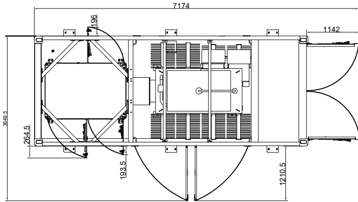
Dimensiones máximas exteriores (Con puertas abiertas)
