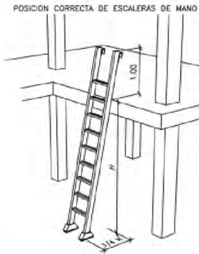
ESCALERA DE MANO
