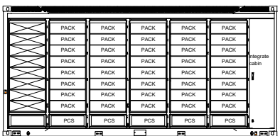
Vista frontal de la extracción del techo
