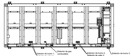
Vista superior (Quitar el panel del techo)
